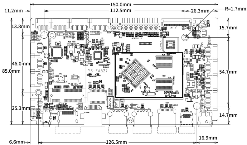
外形尺寸图
