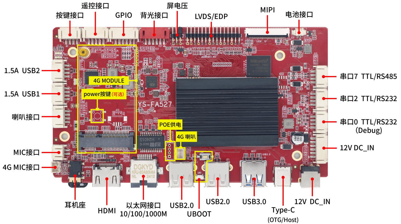
正面接口图
