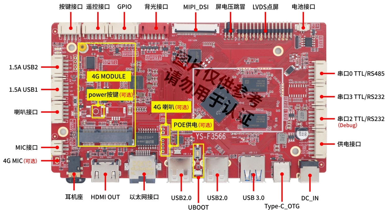
正面接口图
