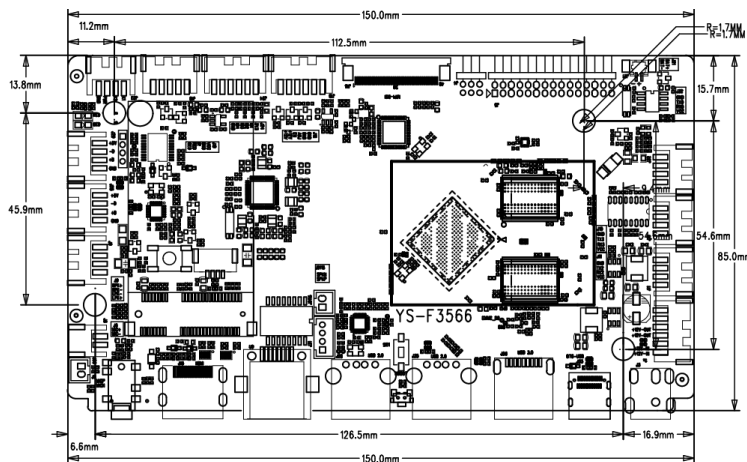
外形尺寸图
